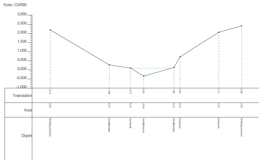
Tværsprofil nr 17
