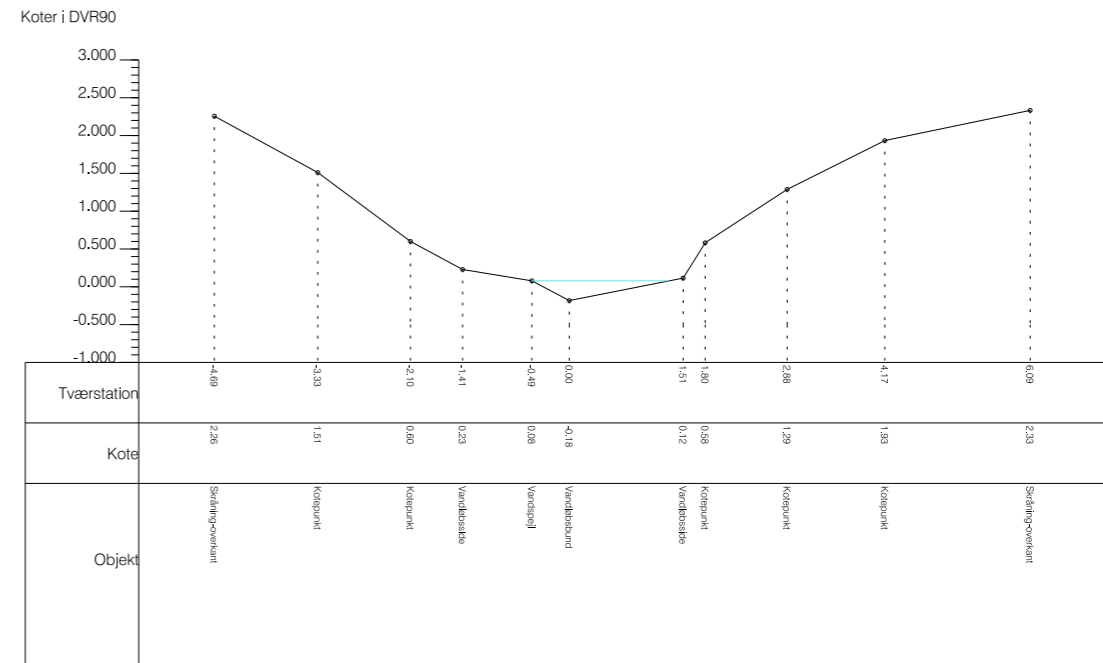
Tværsprofil nr 18
