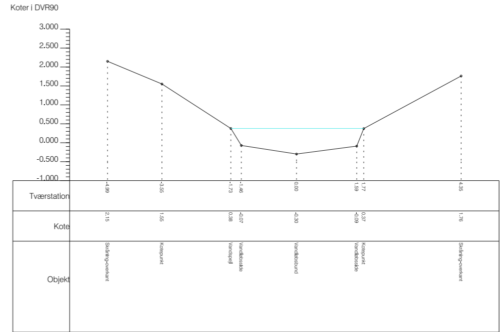
Tværsprofil nr 16
