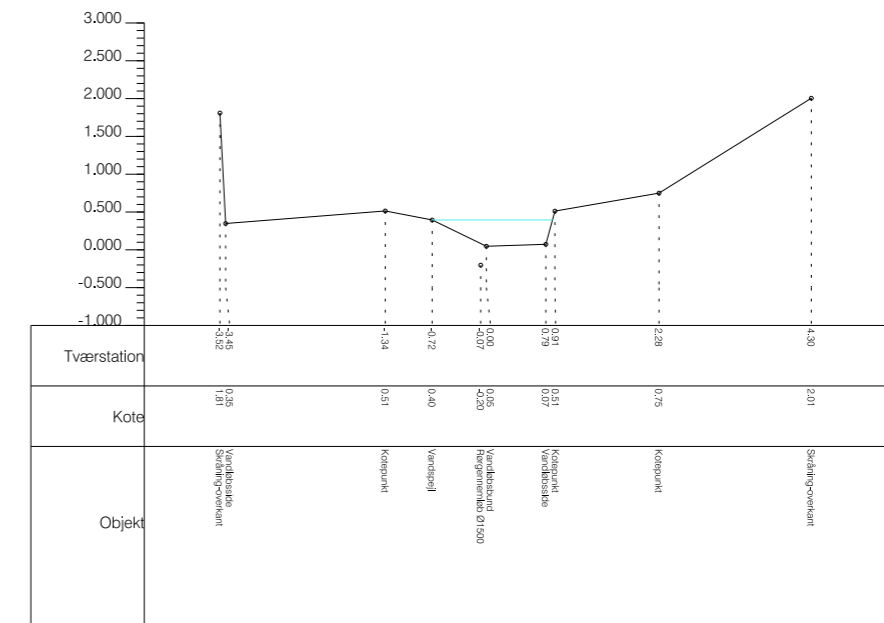
Tværsprofil nr 14
