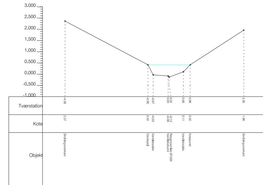
Tværsprofil nr 13
