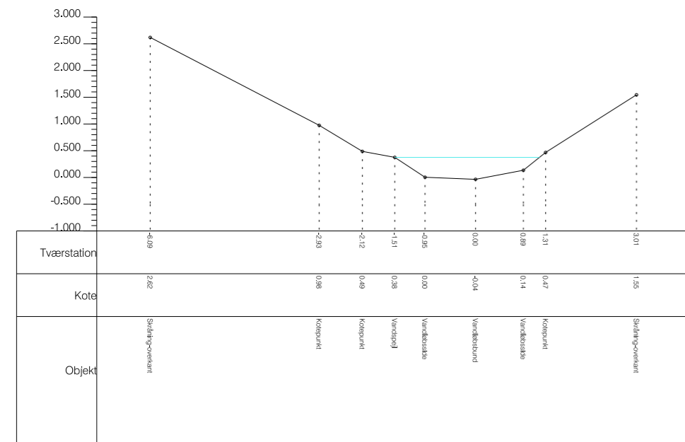
Tværsprofil nr 11
