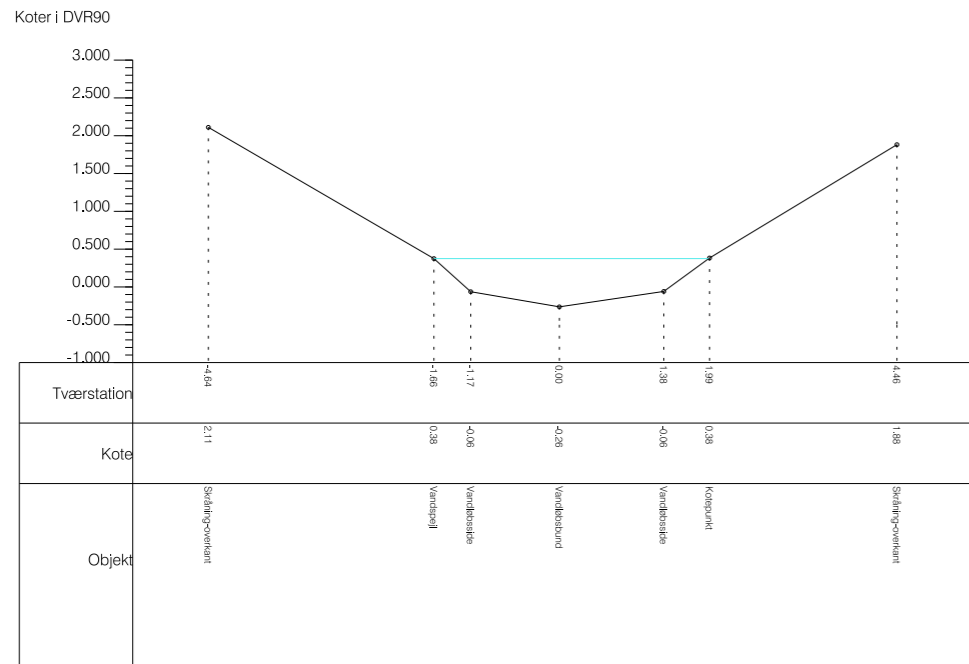
Tværsprofil nr 15
