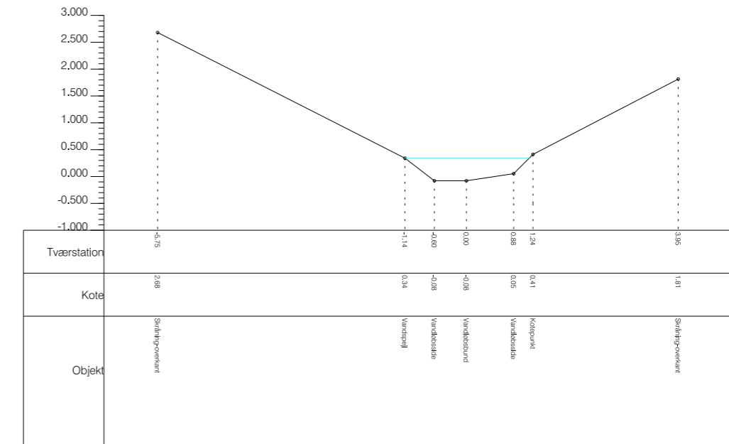
Tværsprofil nr 12
