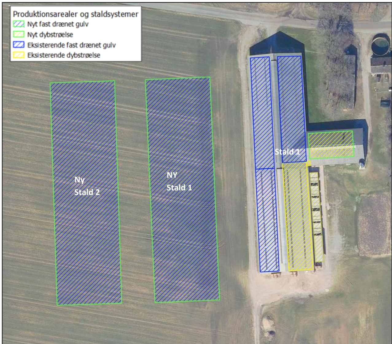
Figur 2. Produktionsarealer for stald 1 og staldstørrelse for Ny stald 1 og 2 (skraveringer) og staldsystemer (farvesymbol).
